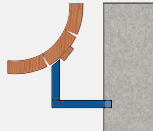
Kastenblende 12 cm wenn keine Nische vorhanden
