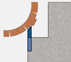
Blende einwärts ab 12 cm Nische
