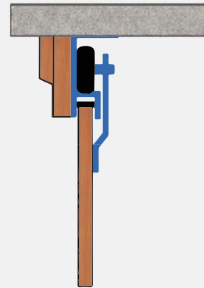
Sturzblende wenn kein Sturz vorhan- den
