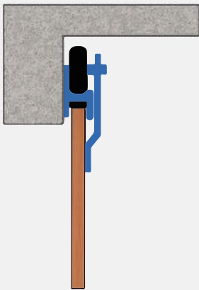
12 cm Normalsturz 10 cm Niedrigsturz
