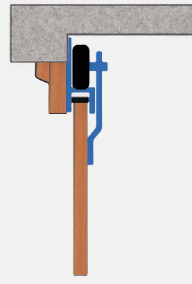
Teilblende wenn Sturzhöhe nicht ausreichend
