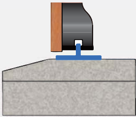
T - Schiene Alu eloxiert auf Estrich aufgebaut
