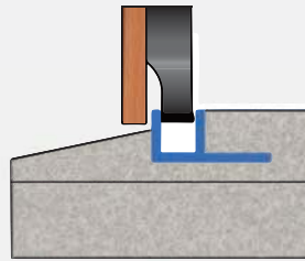
Standardausführung U - Schiene feuerverzinkt oder Edelstahl Nirosta V2A
